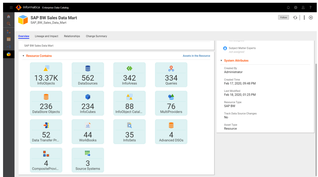
Figura 2: Uma visão geral de todos os objetos que o Enterprise Data Catalog extrai do SAP BW.
